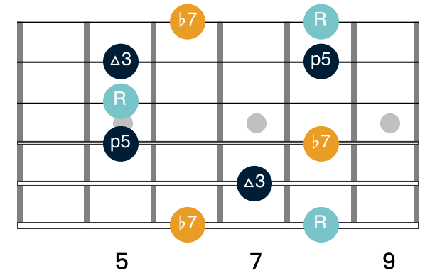
G SHAPE - ARPEGGIO
