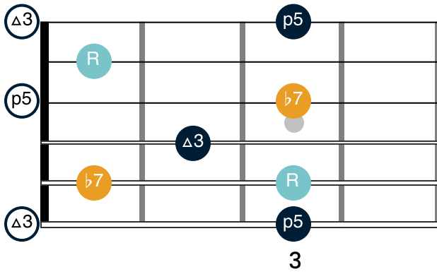
C SHAPE - ARPEGGIO
